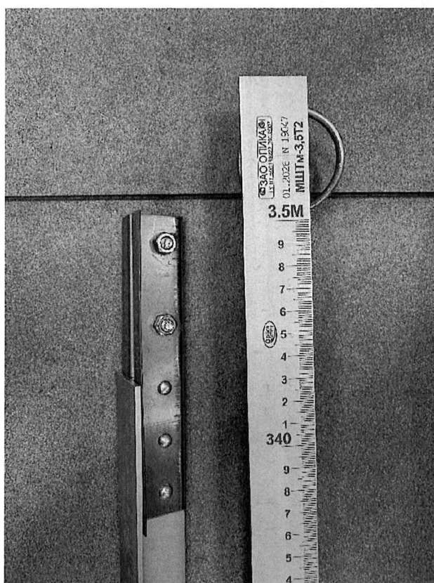
а) Метрошток таврового исполнения
